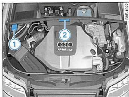
Fig. 267 Compartimento del motor: Datos distintivos del vehículo
