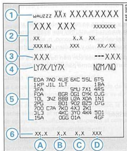
Fig. 268 Portadatos del vehículo
