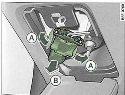
Fig. 265 Desmontar el portalámparas
