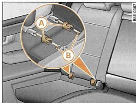
Fig. 190 Argollas de sujeción del asiento para niños ISOFIX
