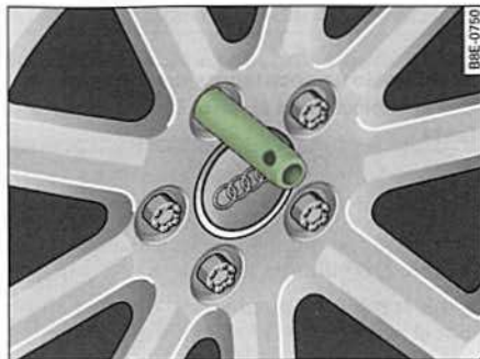
Fig. 237 Cambio de rueda: Pasador de montaje en el agujero superior
