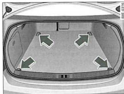
Fig. 97 Disposición de las argollas de amarre en el maletero
