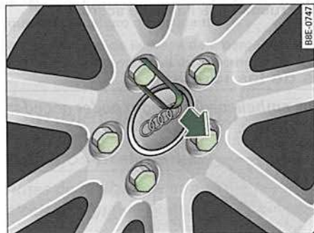
Fig. 232 Cambio de rueda: Quitar las caperuzas de adorno
