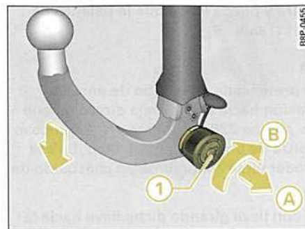
Fig. 203 Dispositivo desmontable para remolque: Desmontar la rótula
