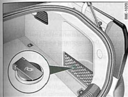
Fig. 116 Detalle del revestimiento lateral del maletero: Toma de corriente de 12 voltios
